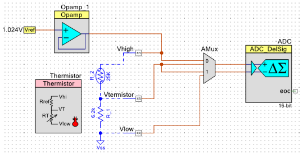
Figura 46: Bloque del convertidor ADC Delta-Sigma para medir la temperatura
