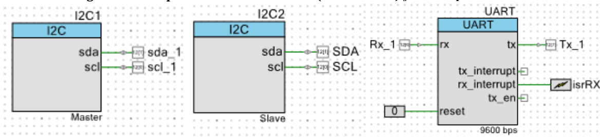
Figura 42: Bloques de comunicación I 2 C (master-slave) y UART para PSOC5
