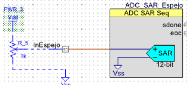
Figura 45: Bloque del convertidor ADC SAR para medir la posición de los espejos
