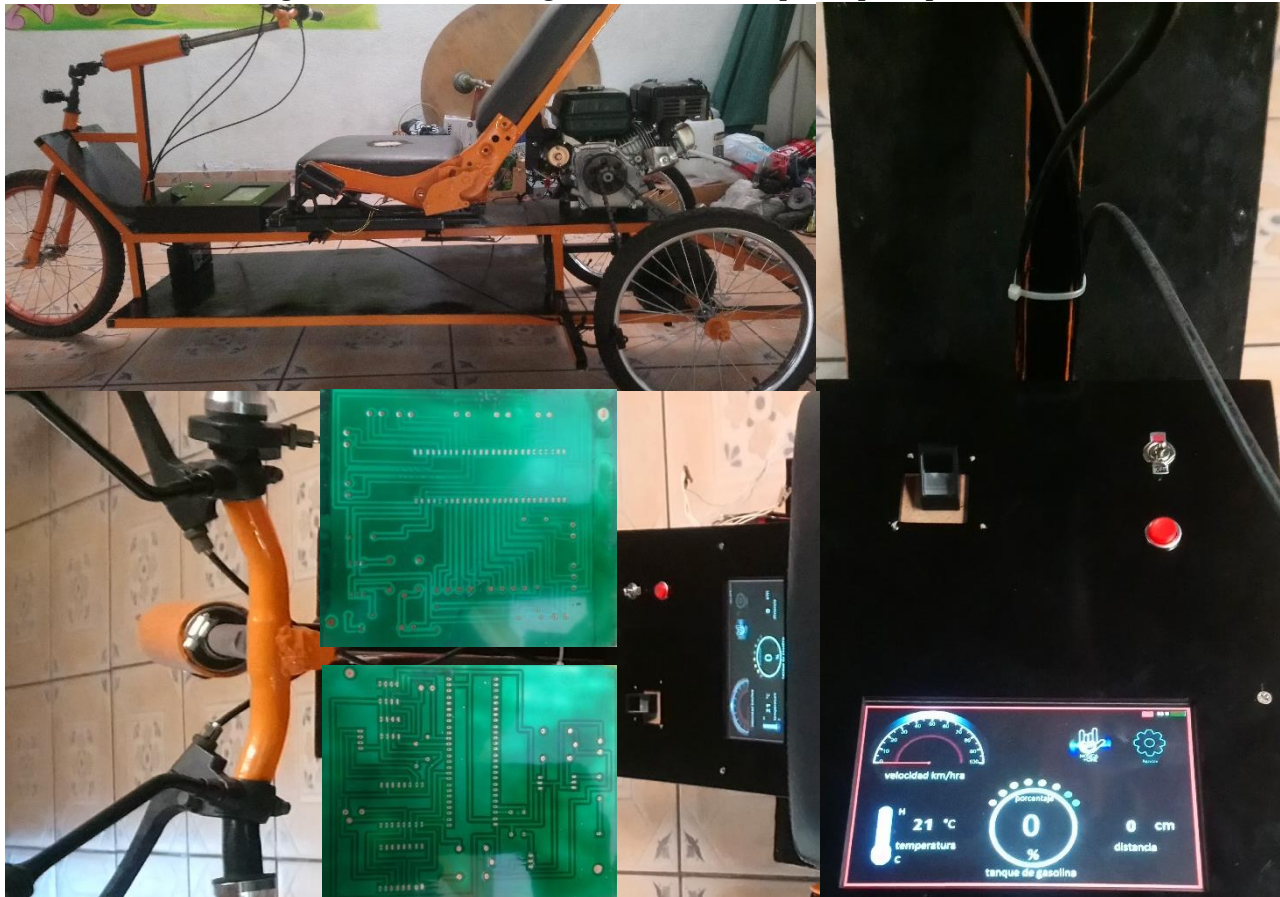
Figura 53: Sistema inteligente instalado en el prototipo de prueba
