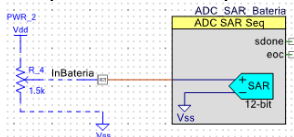
Figura 44: Bloque del convertidor ADC SAR para medir la batería
