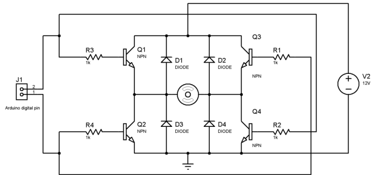
Figura 23: Diseño del funcionamiento de un puente H con transistores
