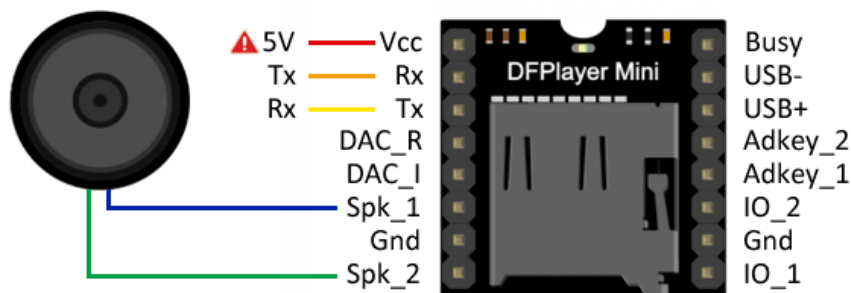
Figura 34: Configuración del módulo MP3 WTV020
