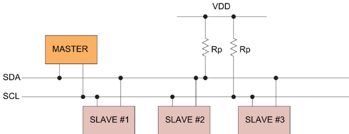
Figura 35: Diagrama del protocolo I 2 C
