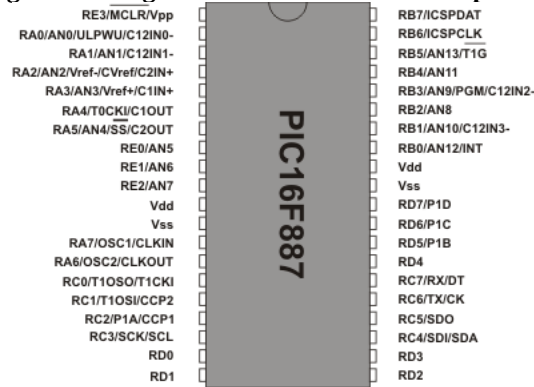
Figura 1: Diagrama del microcontrolador pic16f887
