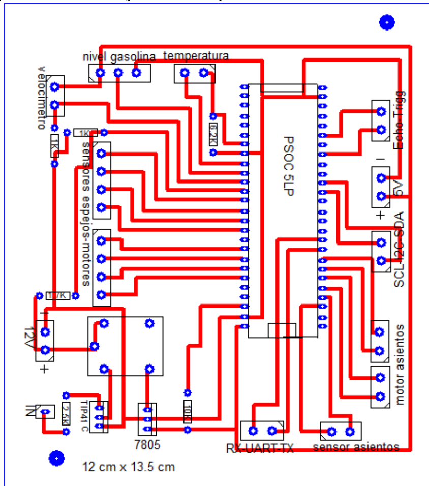
Figura 22: Diseño de tarjeta electrónica para el control maestro de todo el sistema
