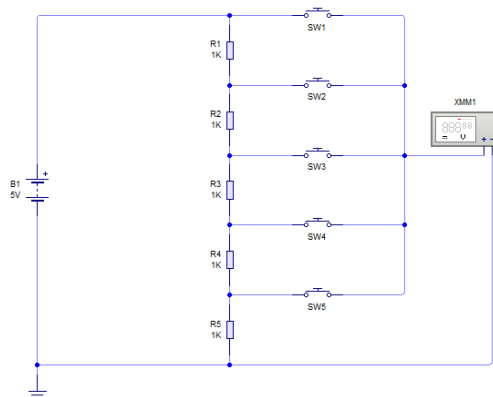
Figura 27: Diseño de divisores de voltajes para las posiciones de los espejos
