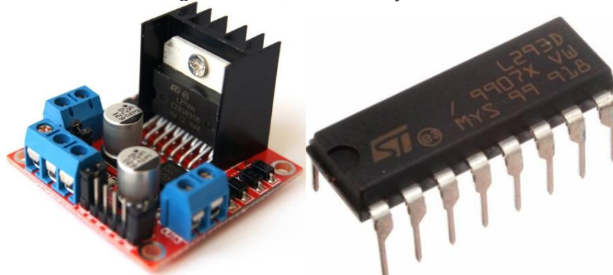
Figura 26: Puente H L298N y L293D
