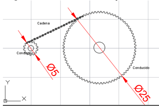
Figura 17: Mecanismo de transmisión por cadena 1:5
