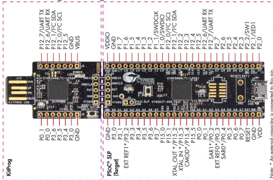
Figura 3: Diagrama del microcontrolador PSOC5
