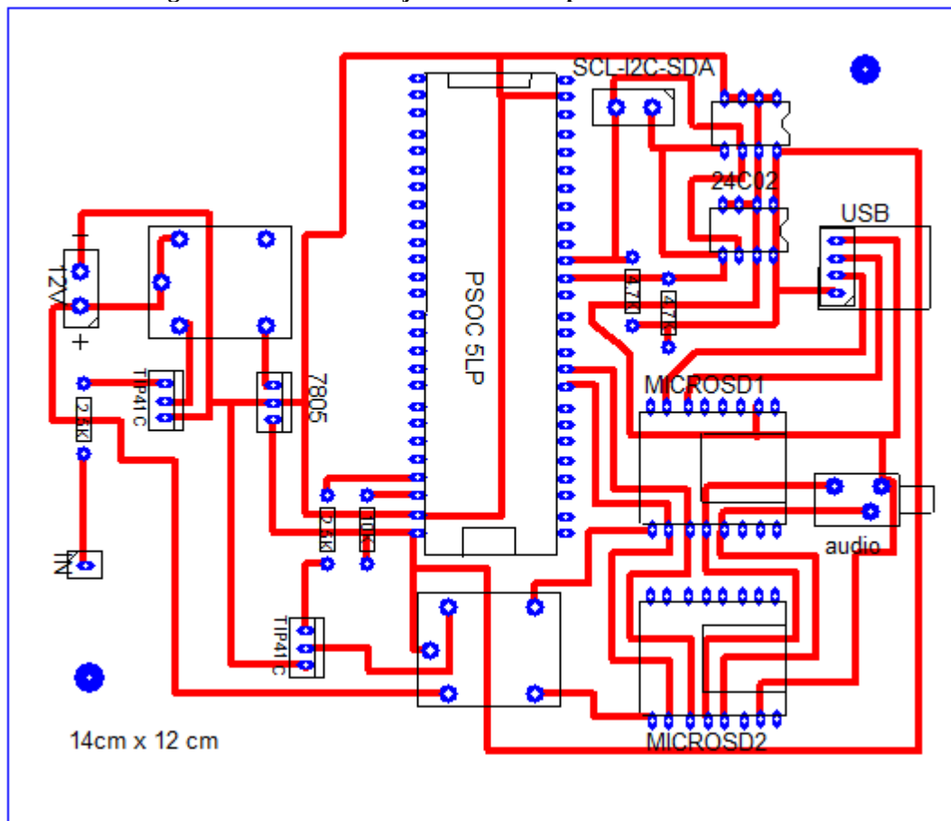
Figura 33: Diseño de tarjeta electrónica para el control de música
