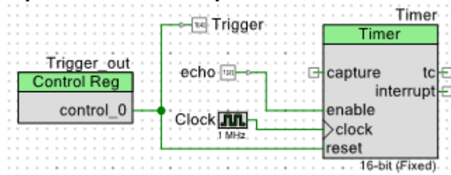
Figura 48: Bloque de control del timer para medir distancias con sensor ultrasónico
