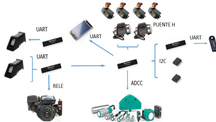
Figura 11: Diagrama de la estructura de comunicación del proyecto
