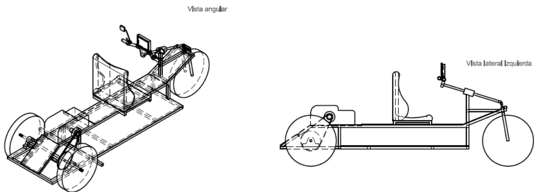
Figura 12: Planos del vehículo go-kart
