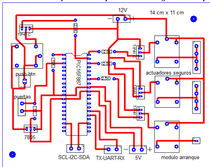
Figura 19: Diseño de tarjeta electrónica para el control de seguridad de las puertas
