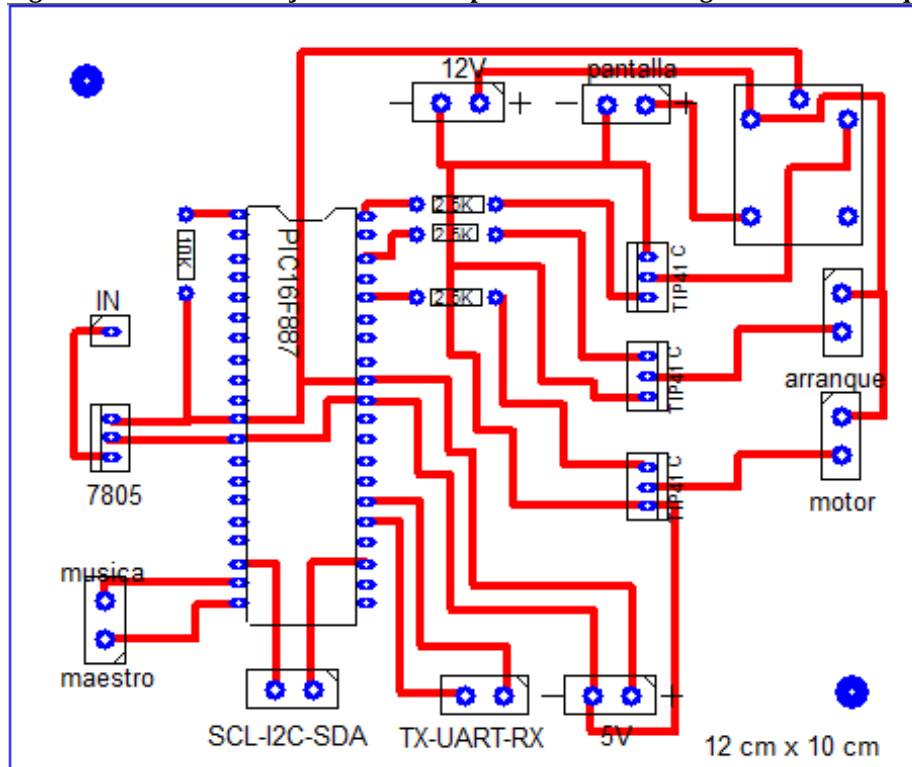
Figura 21: Diseño de tarjeta electrónica para el control de seguridad de arranque
