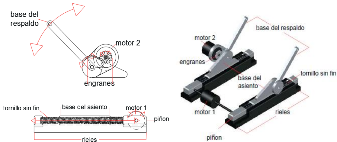
Figura 14: Diagramas de la base del asiento
