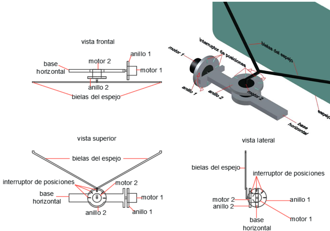
Figura 18: Diseño de mecanismos para el ajuste de la posición de los espejos
