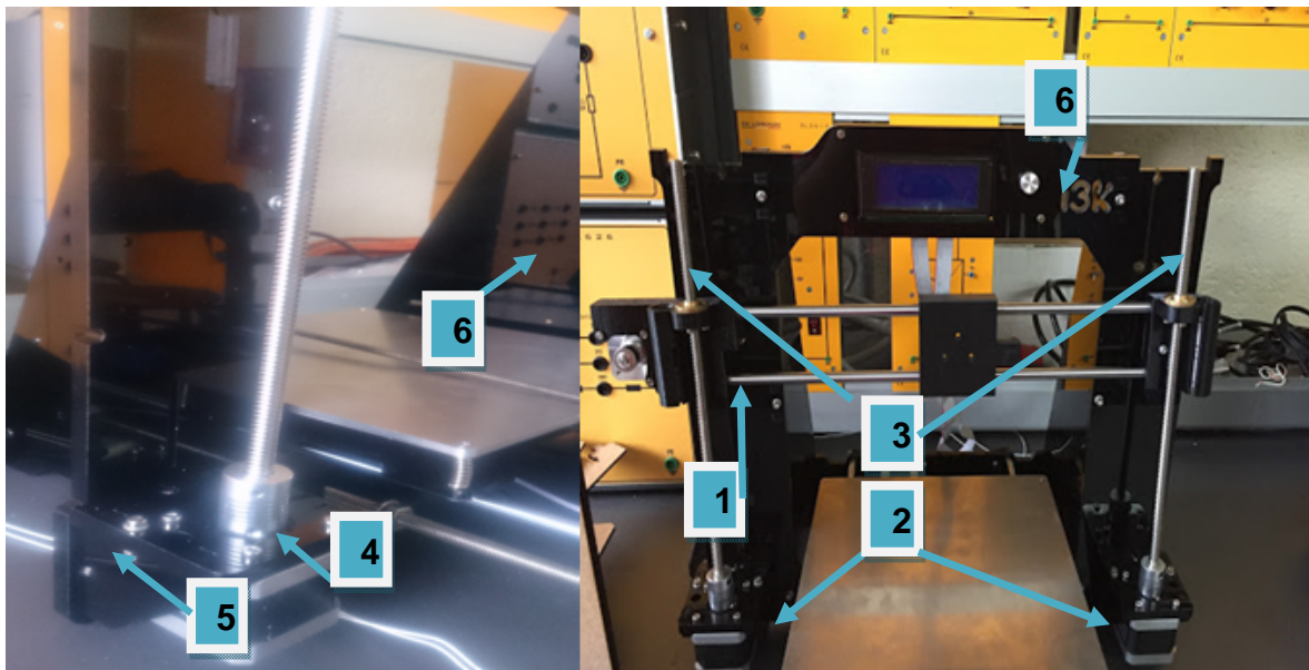
Figura 4.27 Ensamble del Eje Z.
