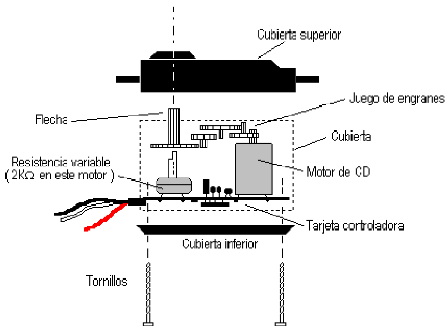
Figura 3.9 Estructura interna de Servomotor CD.
