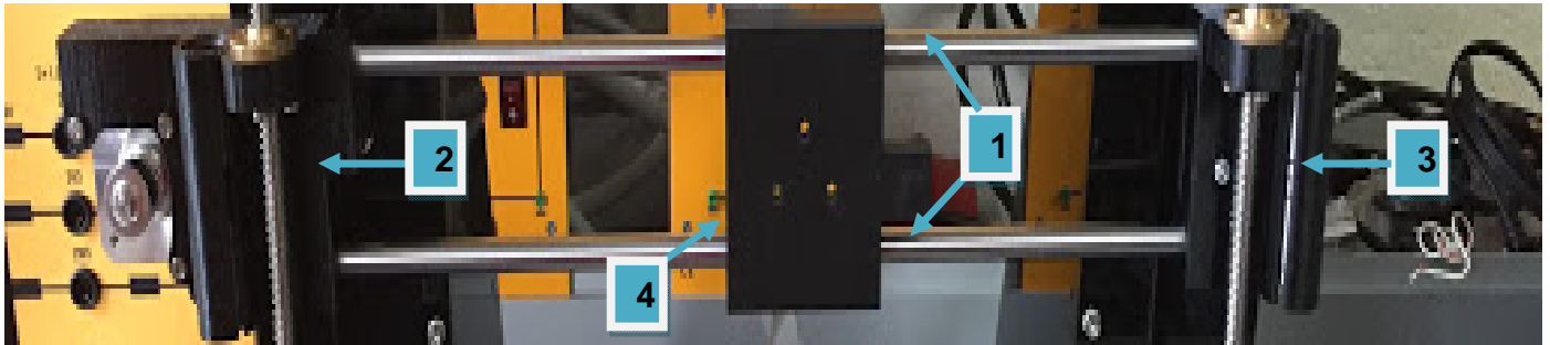
Figura 4.15 Ensamble de Eje X.
