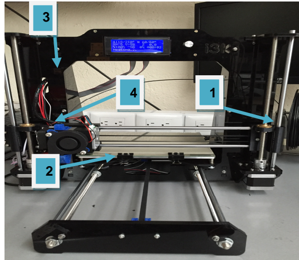
Figura 4.28 Ensamble impresora I3K.
