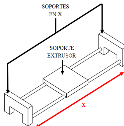
Figura 4.8 Diseño esquemático de Eje X.
