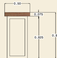
Alzado Lateral
