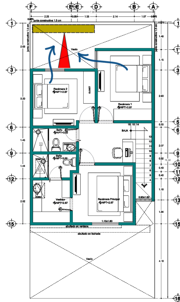
PLANTA ALTA
