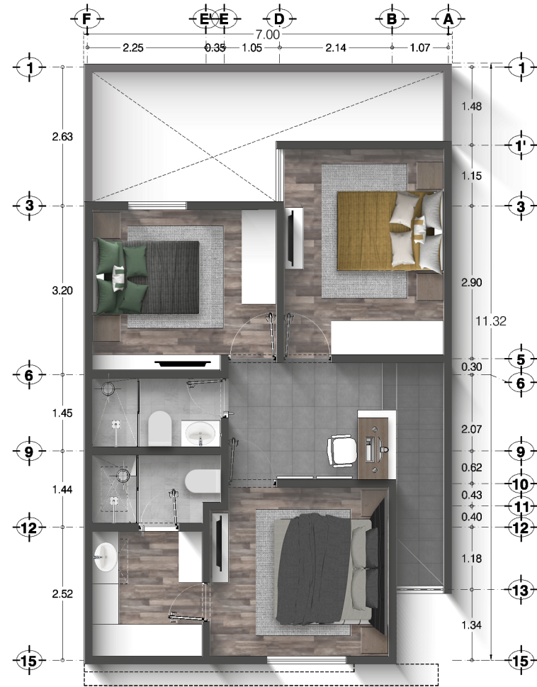
Planta Alta
