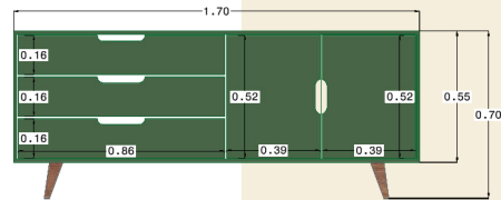
Alzado Frontal
