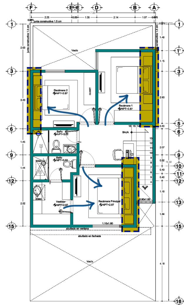
PLANTA ALTA
