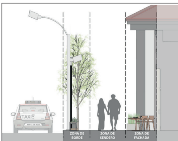
Ilustración 14- Partes de banqueteta (fuente: Norma Técnica de Diseño de calles de Morelia http://semovep.morelia.gob.mx/pdf/normaTecnica.pdf )
